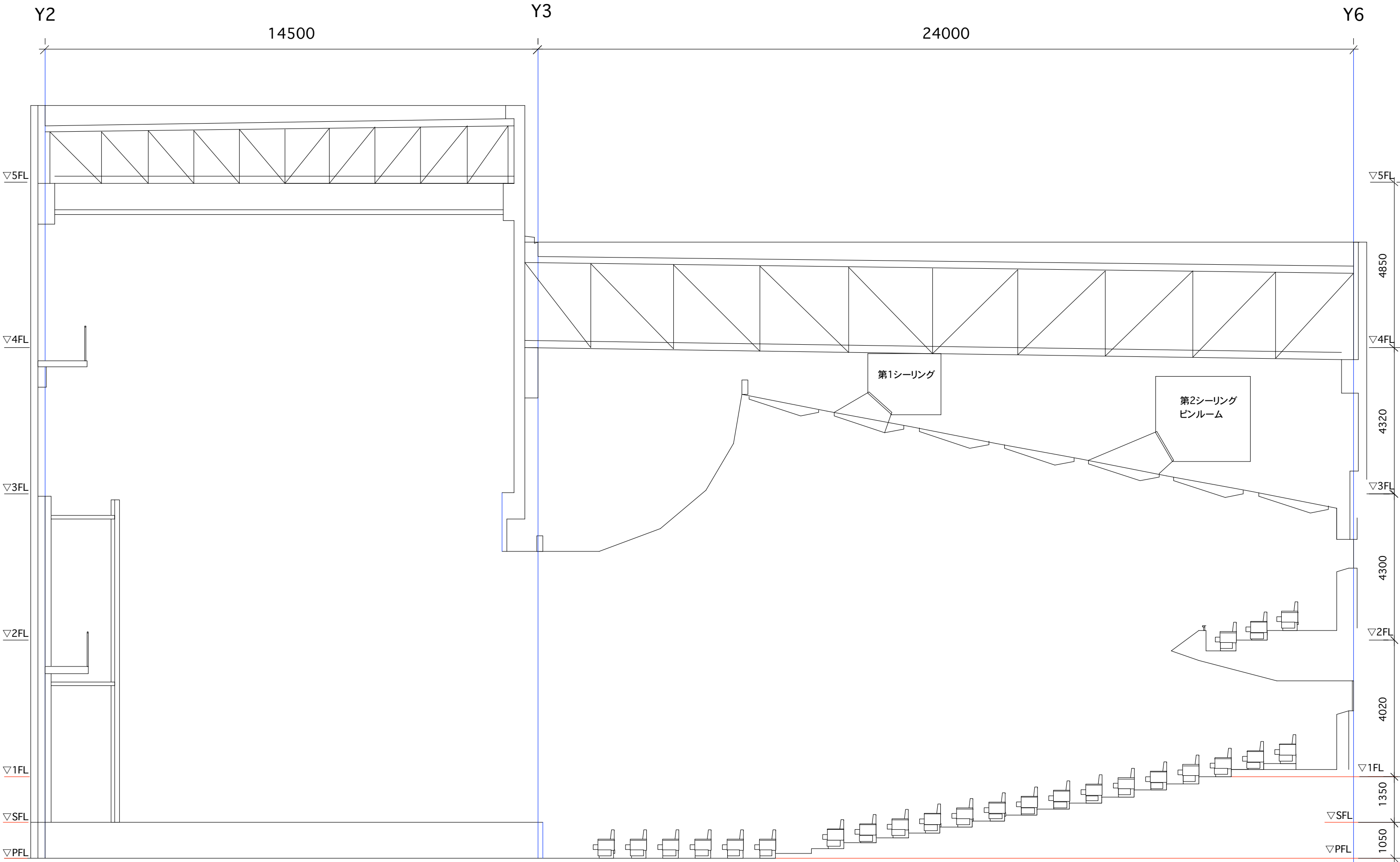
野々市市文化会館フォルテ舞台客席断面図(センター)
