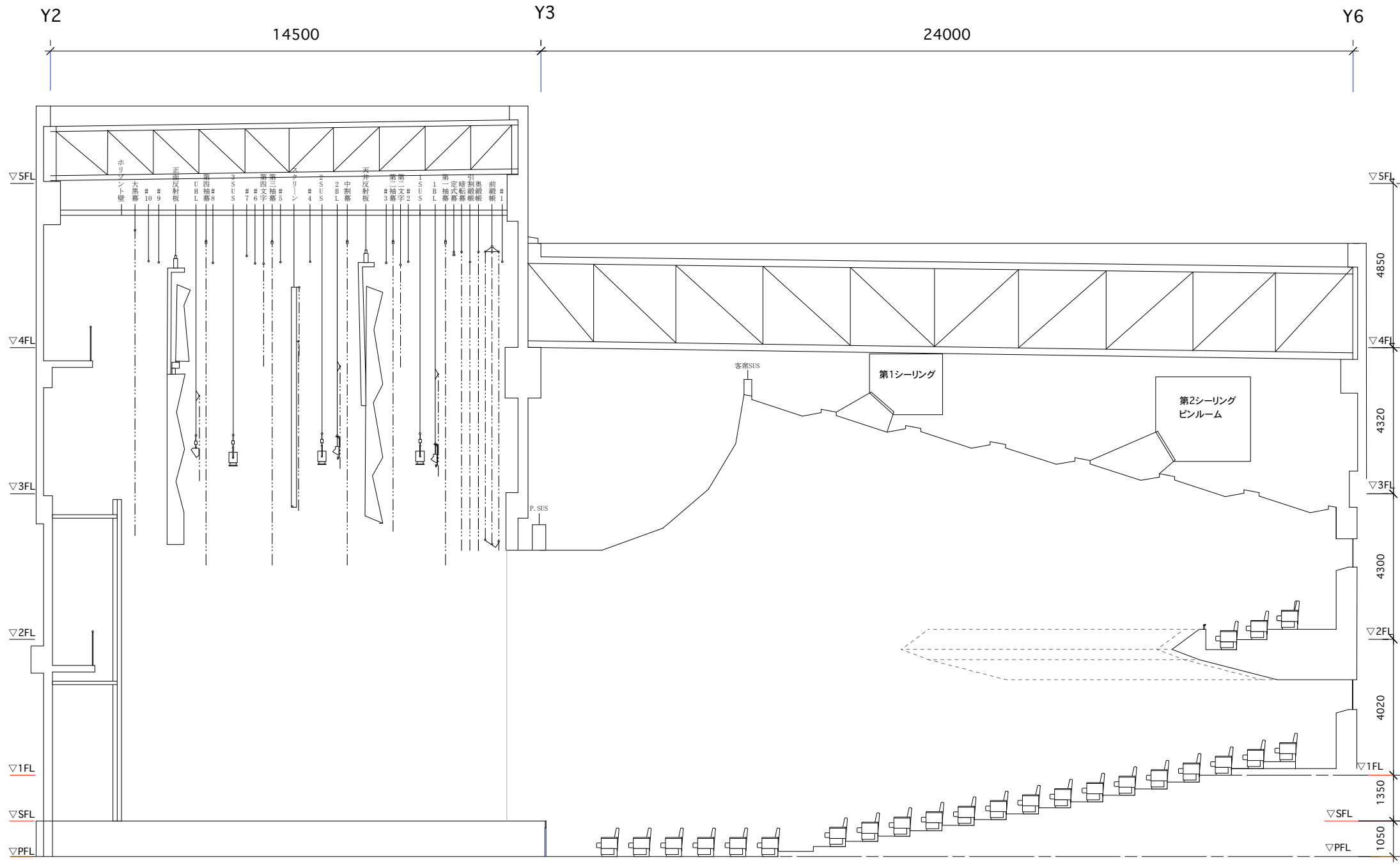
野々市市文化会館フォルテ大ホール 断面図(中央)
